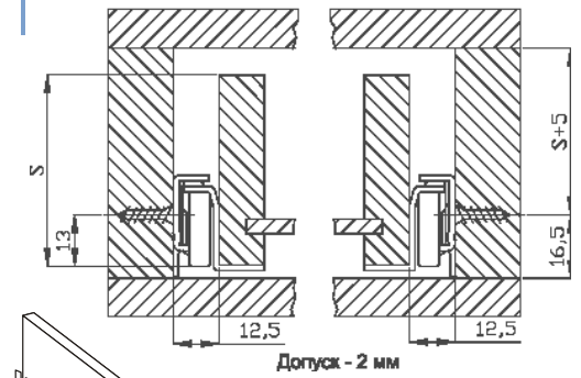
Схема установки направляющих ящика
