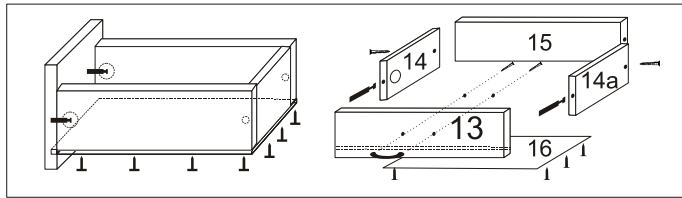
Сборка ящиков
